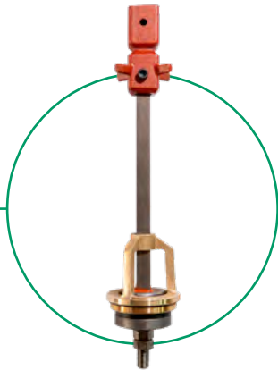
<HIDN100CO Detalle del Conjunto obturador HIDRANTE COLUMNA
