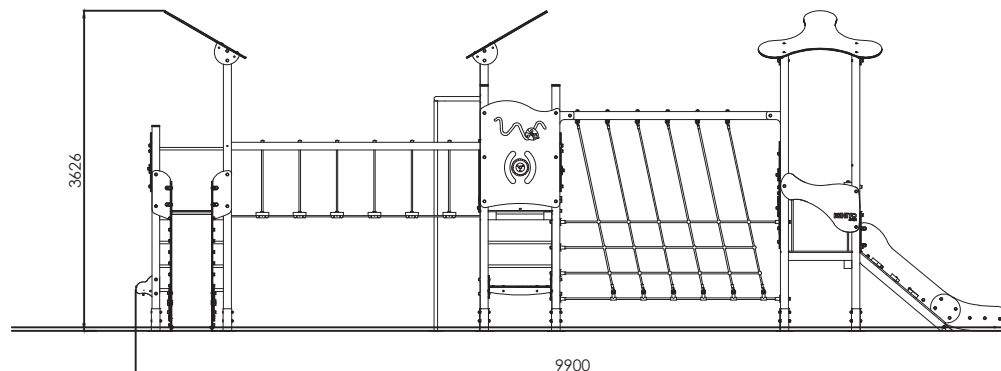
ALZADO
